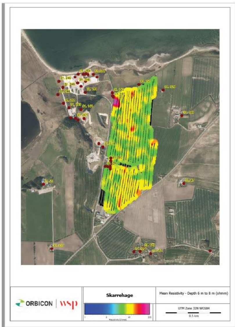
Middelmodstandskort fra kortlægningen i dybden 6-8 meter. Kortet viser, at der på hele matriklen findes moler (gule og grønne farver modsvarer molerets modstand målt i ohmm).
