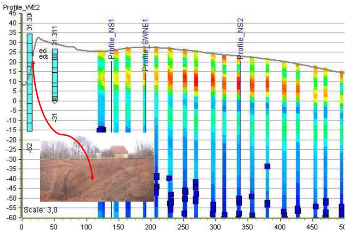
Vest-øst gående profil, der viser molerets udbredelse i dybden. Den øverste orange farve indikerer overjord/muld. De grønne, gulorange og røde farver nedenunder viser molerets udbredelse i dybden.
